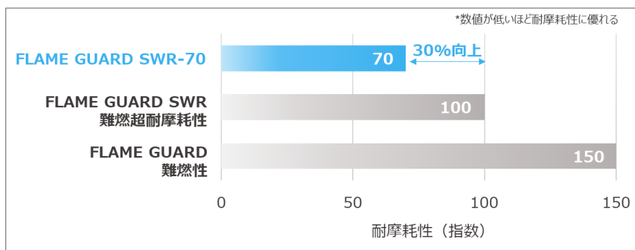
「FLAME GUARD」シリーズの耐摩耗性比較
