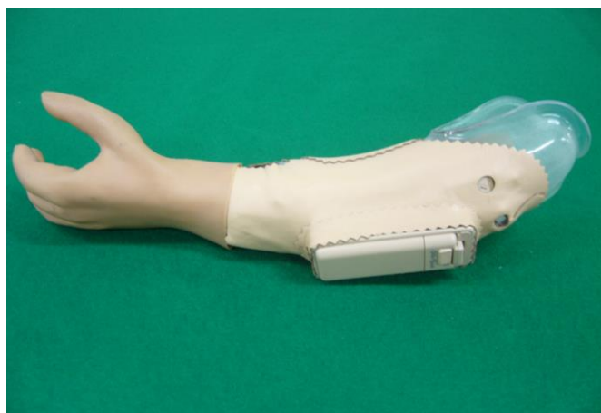
本人の意思で指を動かせる筋電義手
