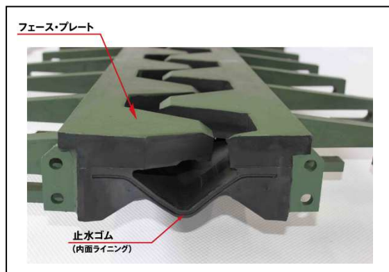
YHT-N 型の製品断面
